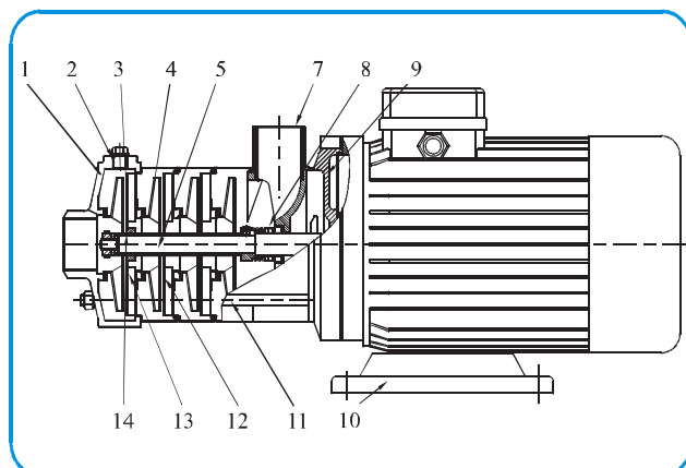
截面图 CHLF,CHLF(T)
