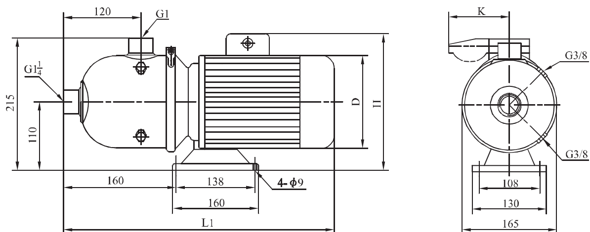
安装图
