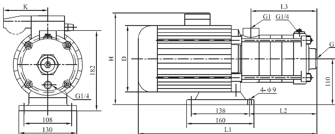
尺寸和重量
