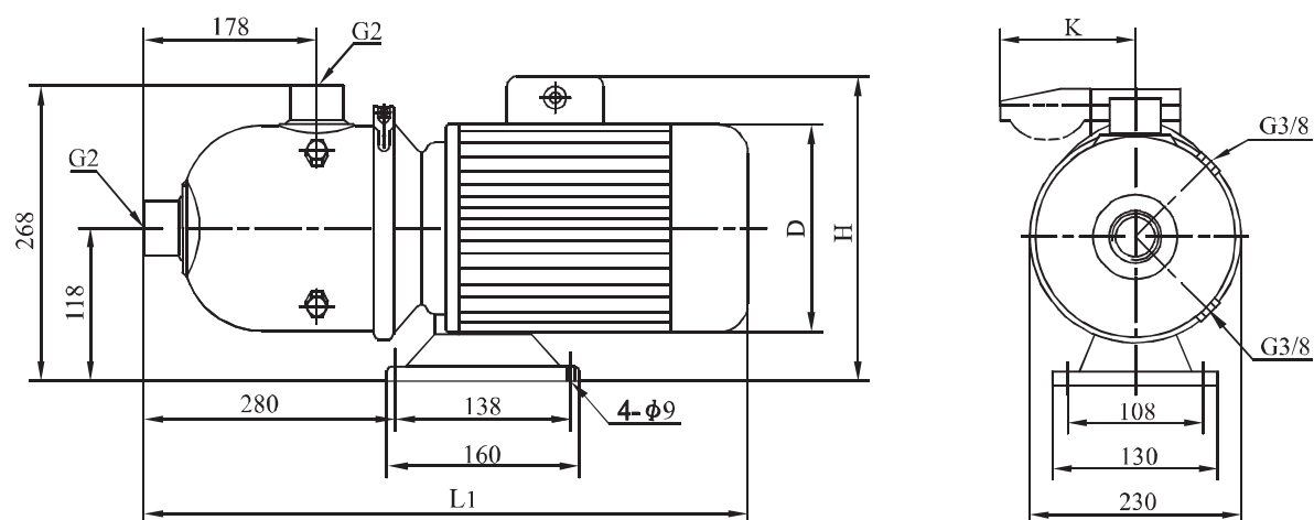
安装图
