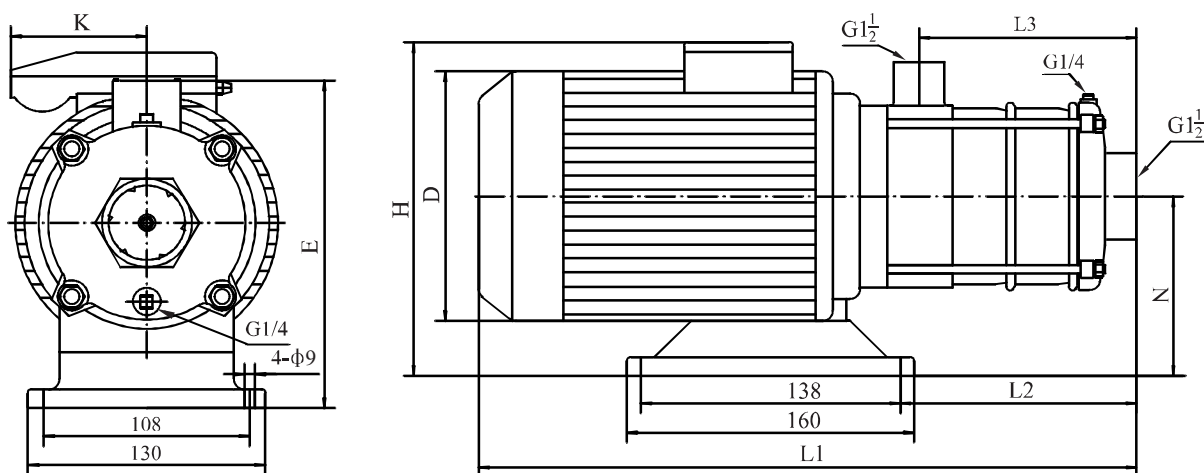
尺寸和重量
