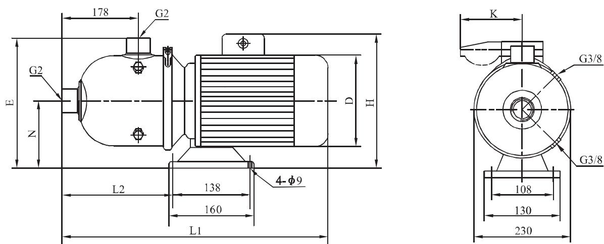
安装图
