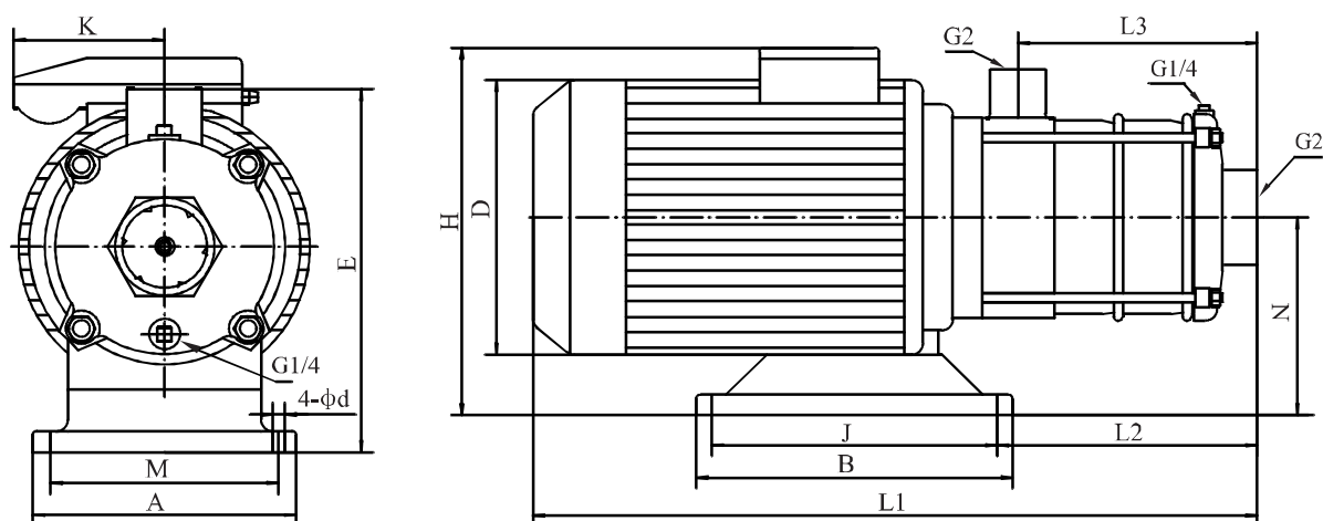
尺寸和重量
