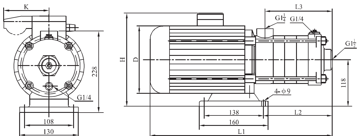
尺寸和重量
