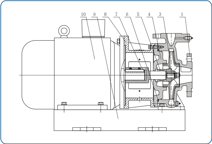
NIS, NISF零件材料
