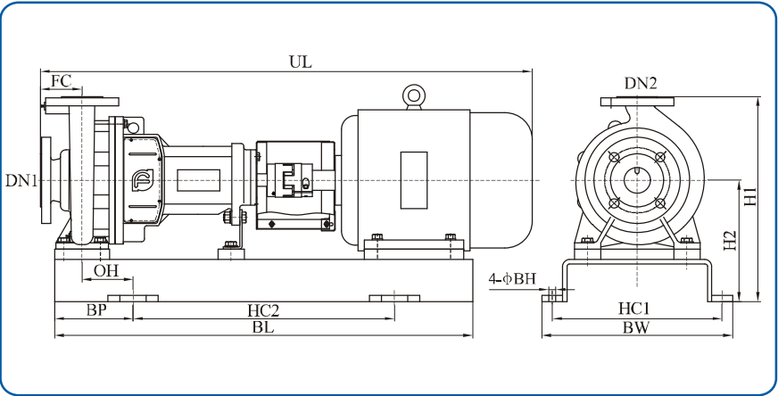
NISO泵组外形尺寸表
